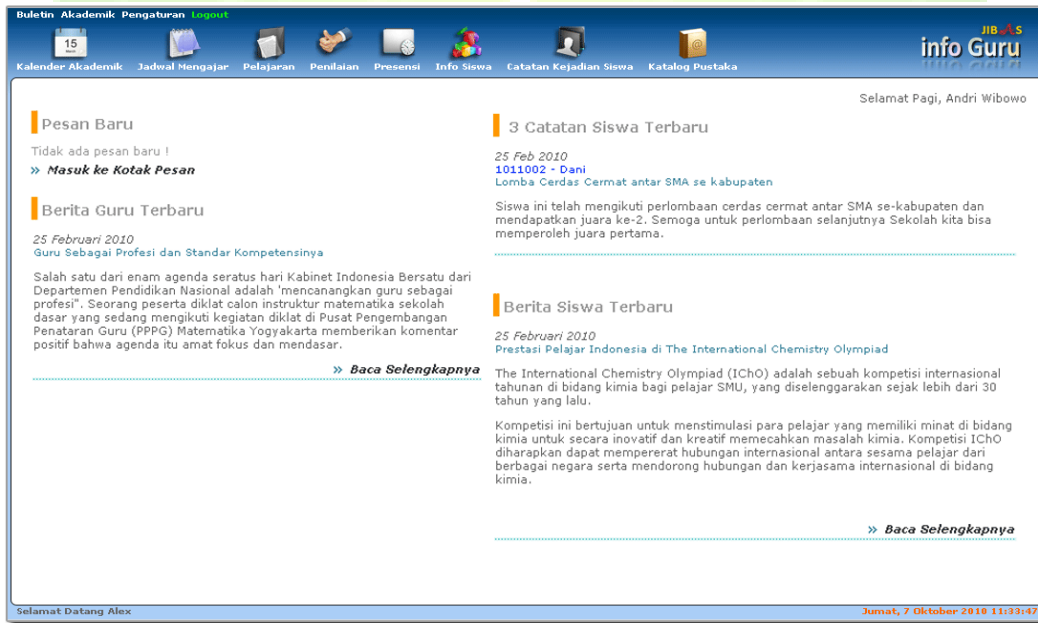
Gambar 23. Menu Akademik
