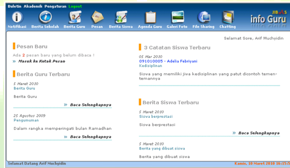
Gambar 2. Menu Buletin
