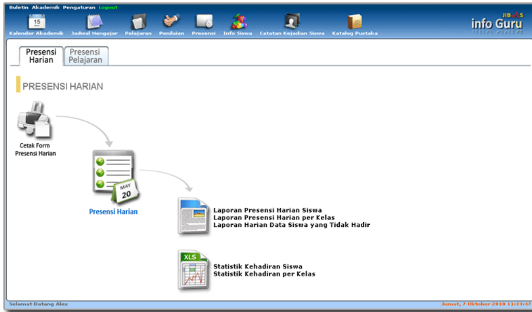
Gambar 50. Menu Presensi
